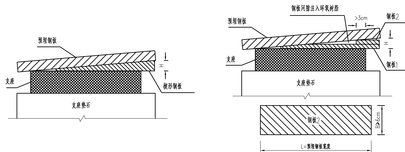
楔形钢板A大样
