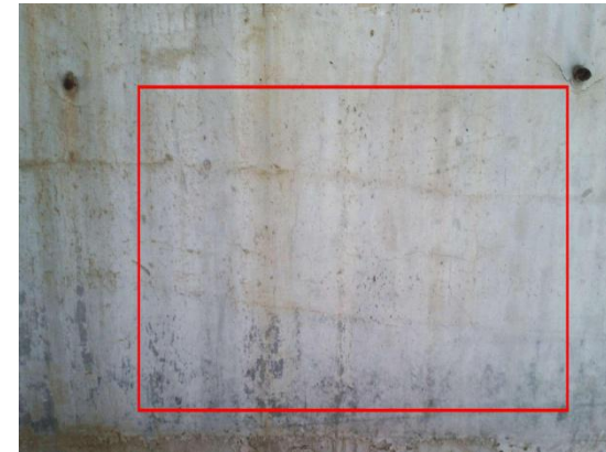
图 3-8: 元潭 2 号大桥右幅 GL-R-5D 盖梁: 距右侧 1m 处, 大桩号面网状裂缝; 数量: 1 条, 长度: 1.0m, 宽度: 1.50mm。
