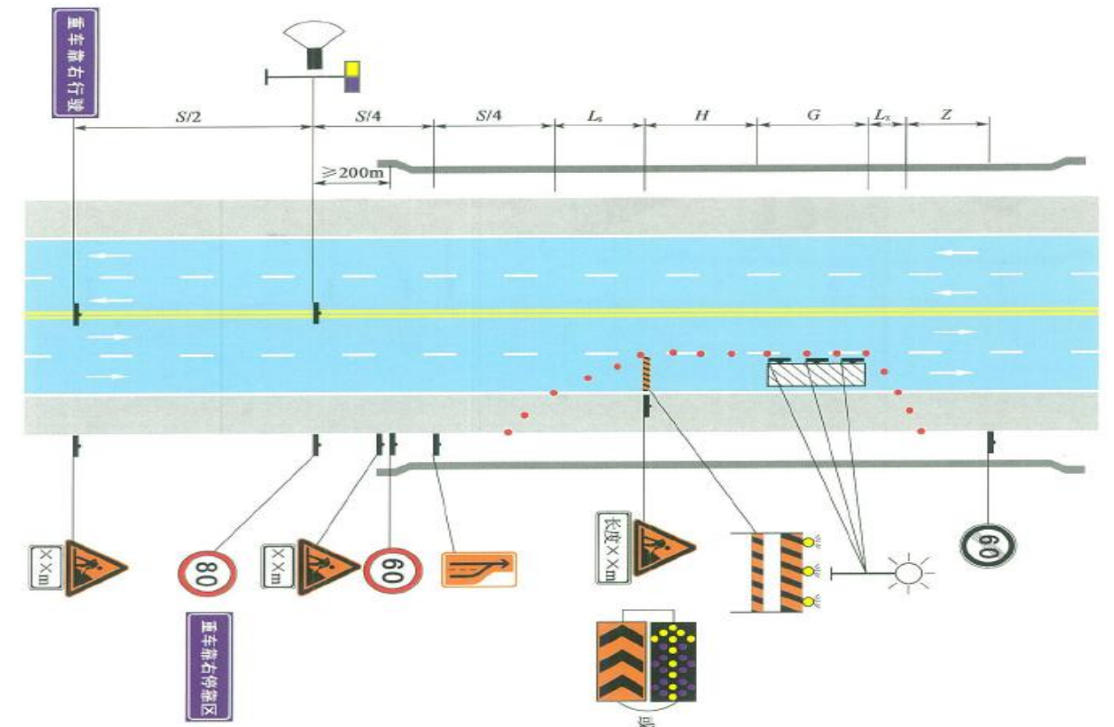
图 8-2 工作区起点距桥头大于或等于 300m 的特大、大桥封闭车道养护作业
