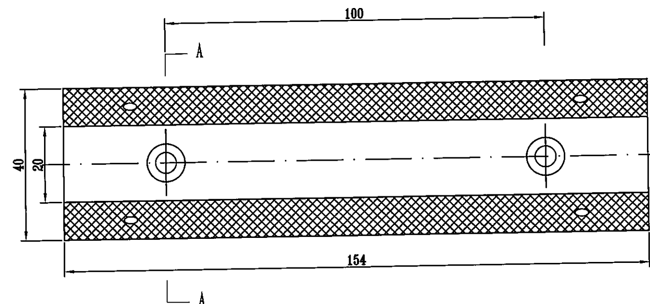
De-Rby(Rbw)-At3立面图 1:1
