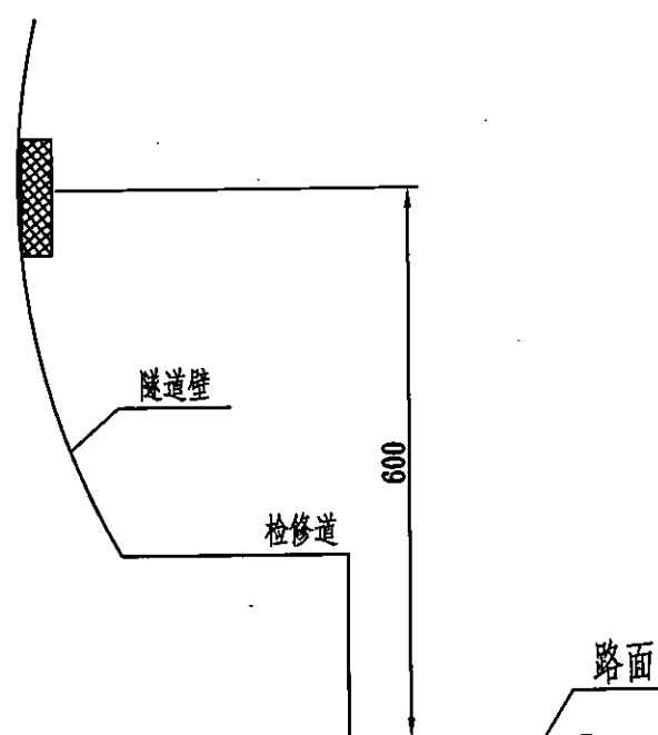
De-Rby(Rbw)-At3安装示意图
