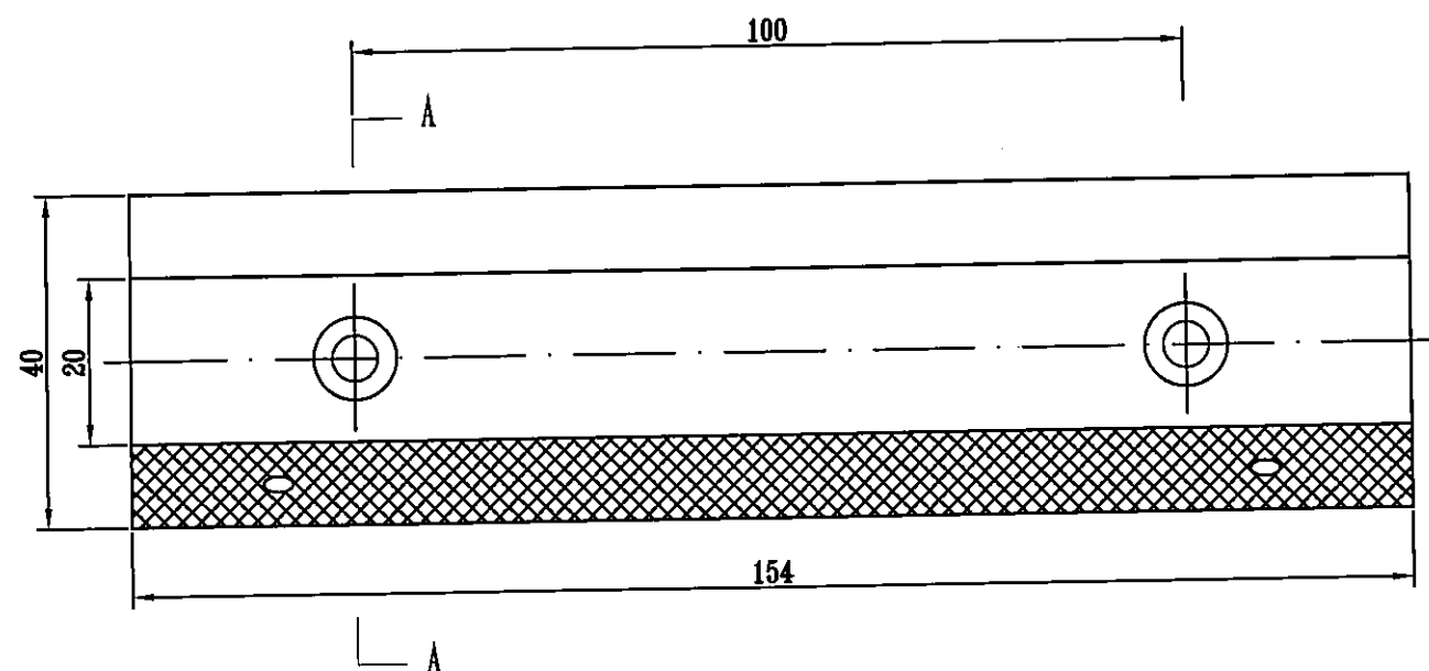
De-Rby(Rbw)-At2立面图 1:1
