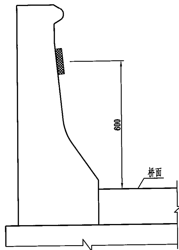
De-Rby(Rbw)-At2安装示意图
