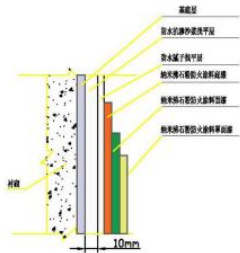
隧道壁涂料喷涂大样图
